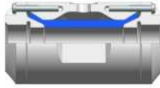
FOT. 9, 10 Przekrój przez zawór kołnierzowy (po lewej) i przekrój przez zawór gwintowany
